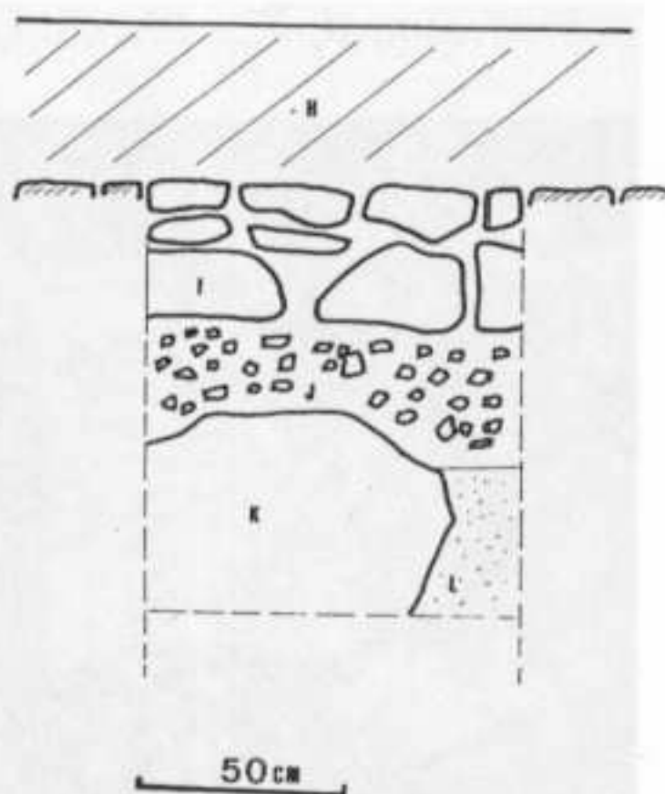
Fig. 5 - Coupe des fondations du bâtiment B
