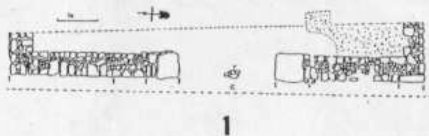
Fig. 6 - Position respective des deux départs de bâtiments B et C du plan de masse
