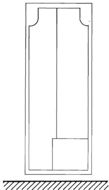
PL. VII - Intérieur, latrines du 1 er étage : plan, coupe et élévation, par P. Roques.
